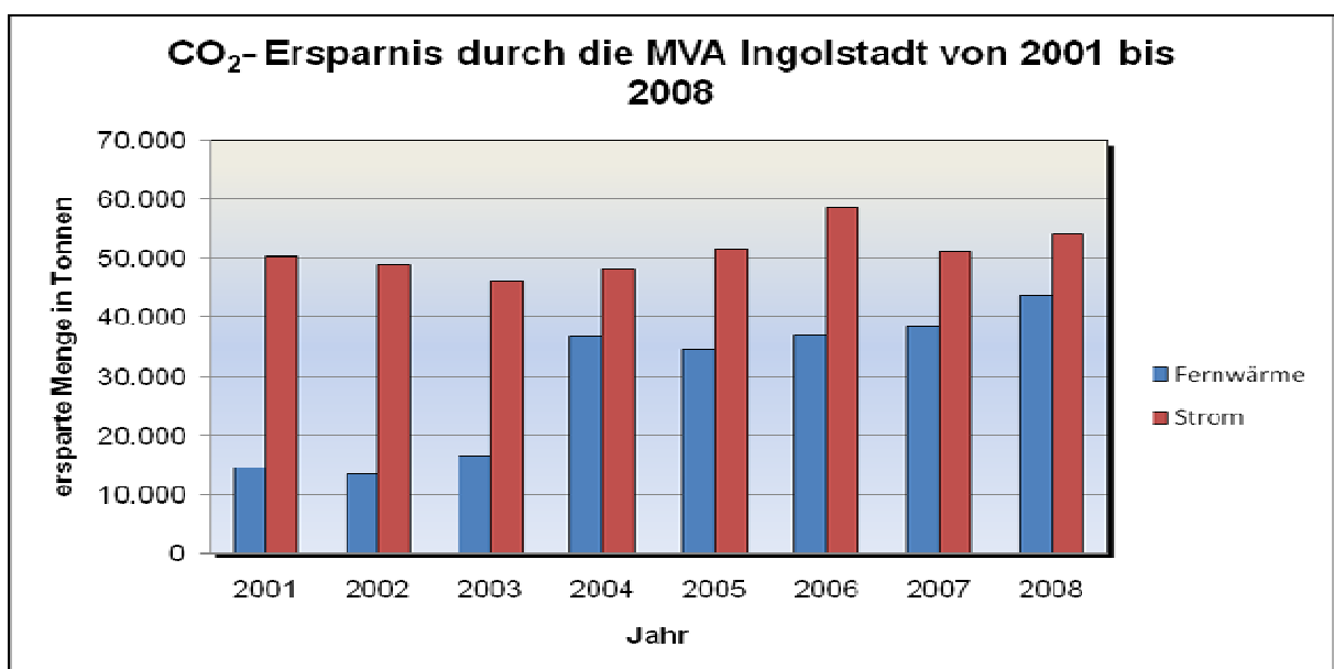
Übersicht 6: CO 2 -Ersparnis durch die MVA Ingolstadt von 2001 bis 2008
