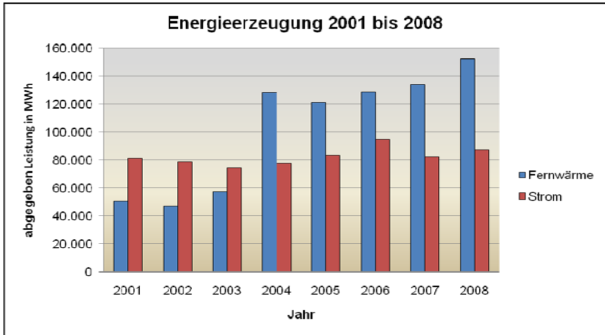
Übersicht 5: Energieerzeugung 2001 bis 2008
