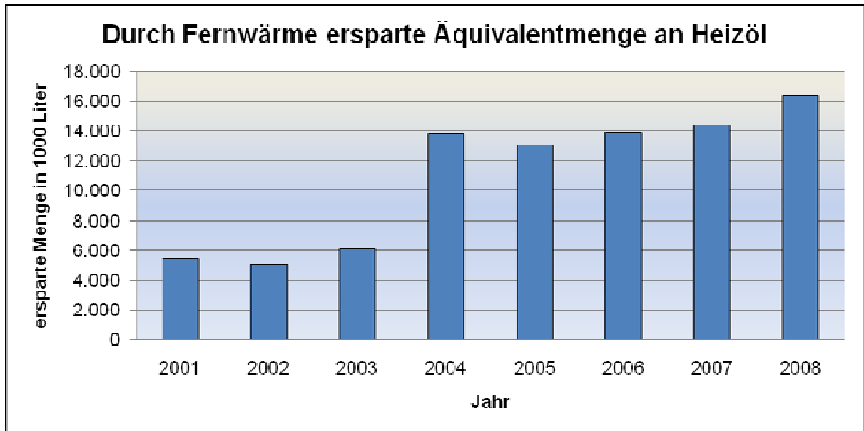
Übersicht 7: Durch Fernwärme ersparte Äquivalentmenge an Heizöl EL von 2001 bis 2008
